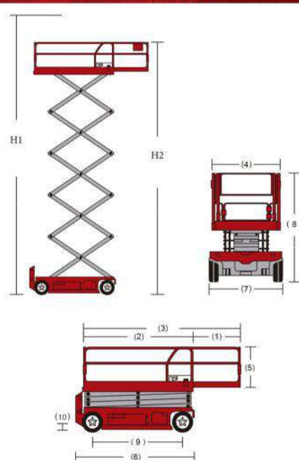
Diagrama de dimensiones del equipo
