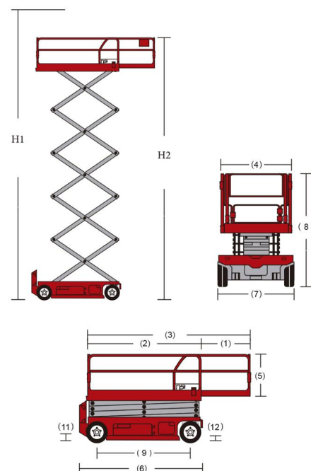
Diagrama dimensiones
